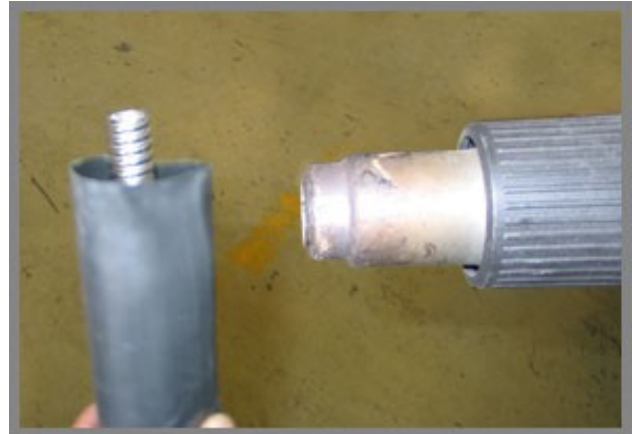
Schrumpfschlauch aufstecken
